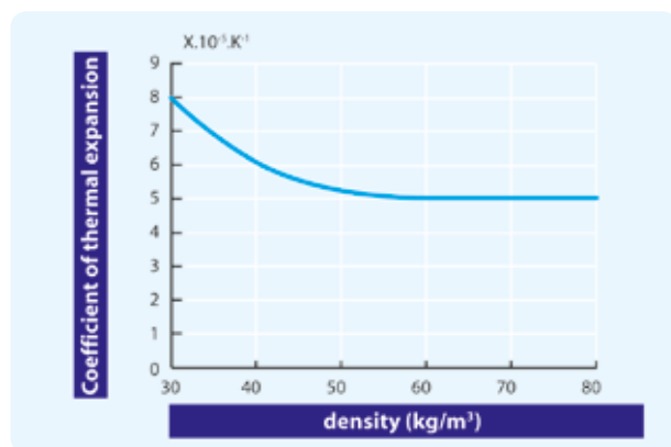
Bilde 8: Varmeutvidelsen til stivt polyuretanskum (PUR/PIR) uten dekklag. (Varmeutvidelsen til stivt polyuretanskum (PUR/PIR) uten dekklag i temperaturer mellom -60 °C og +20 °C, målt i forhold til tetthet)
